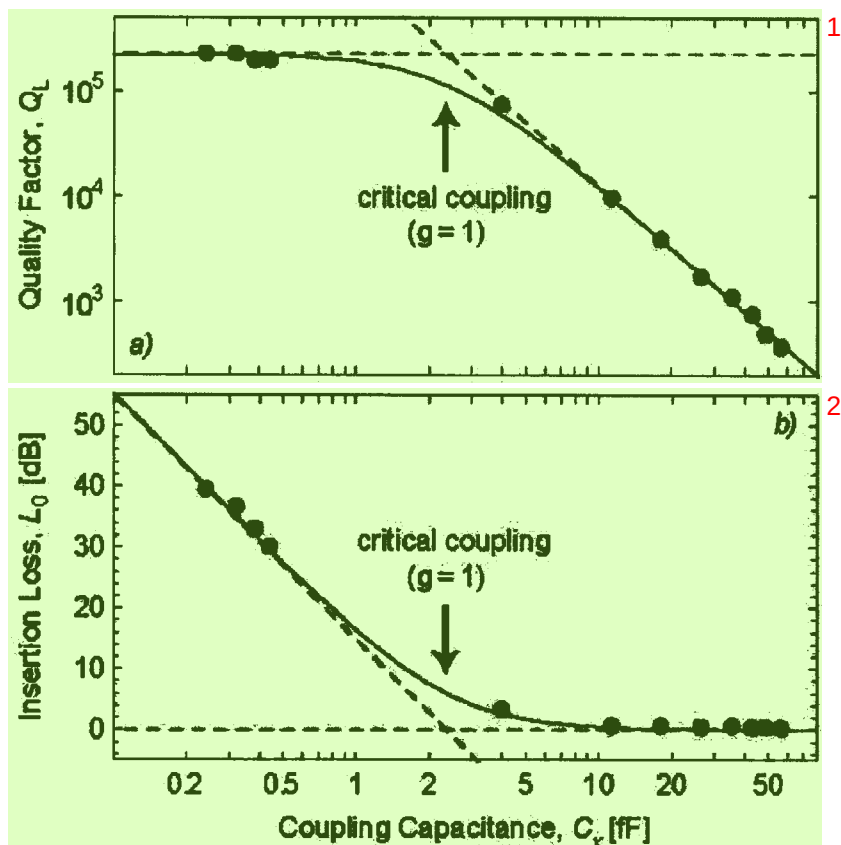
图 3.7 有载品质因子和插入损耗随耦合电容的变化 [50]
