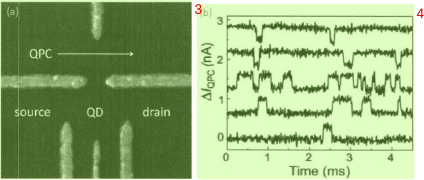
图 1.11 (a)QPC 结构 (b) 使用 QPC 测得的量子点中电子隧穿信号 [15] 5
