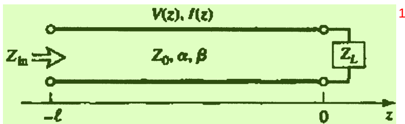
图 3.2 传输线模型
