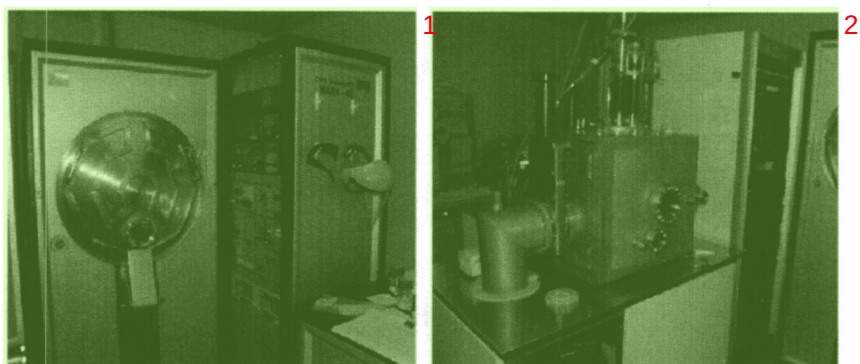
图 2.5 电子束镀膜机和热蒸发镀膜机 3
