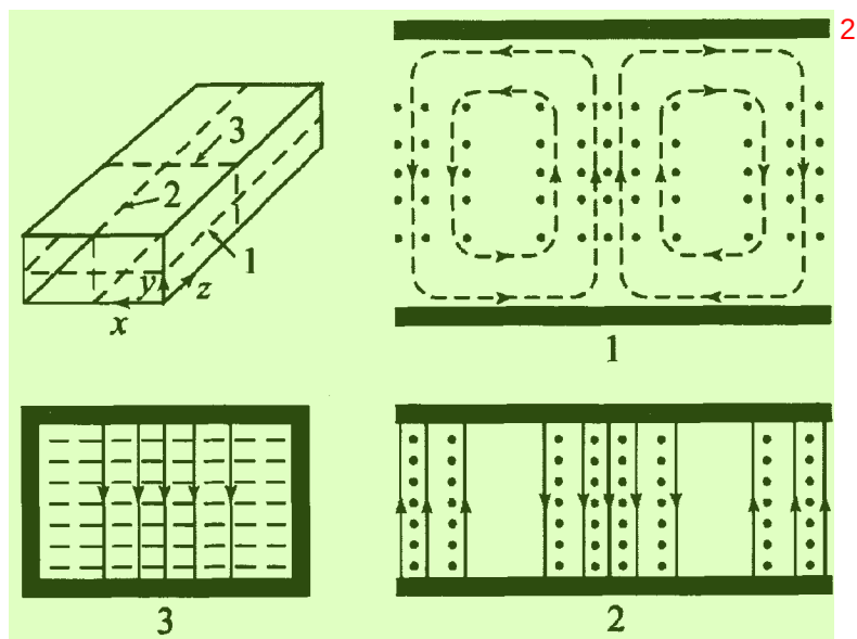
图 3.19 TE_{10} 模电磁场分布 [48]
