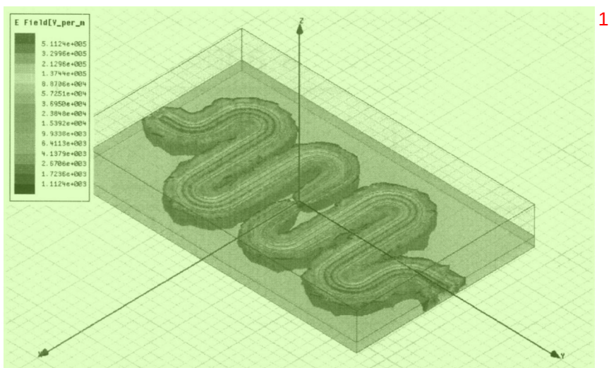
图 3.9 透射式谐振腔电磁模拟
