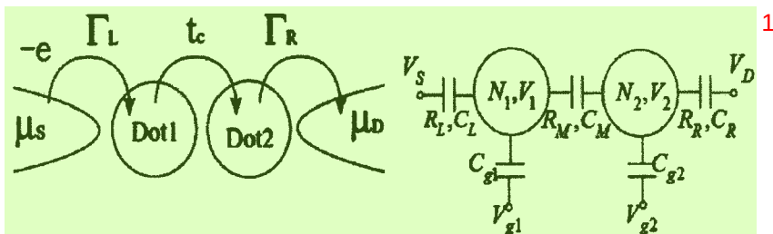
图 1.6 双量子点常相互作用示意图
