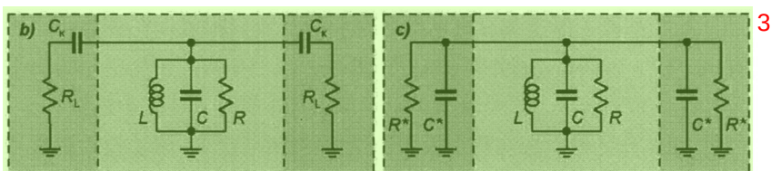
图 3.6 透射式谐振腔等效电路 [50] 4
