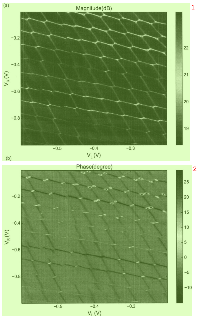
图 5.2 (a) 谐振腔反射谱振幅随控制门电极 L 和 R 变化。六边形蜂窝形状是双量子点输运相图的典型图样 (b) 相同电压区域谐振腔相位的变化
