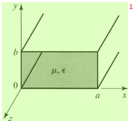
图 3.18 矩形波导结构 2
