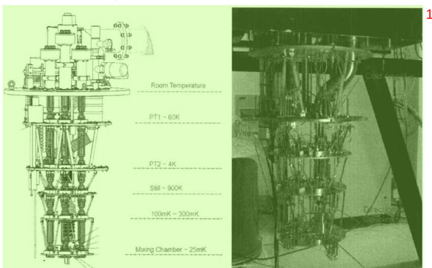
图 2.12 稀释制冷机示意图和实际结构
