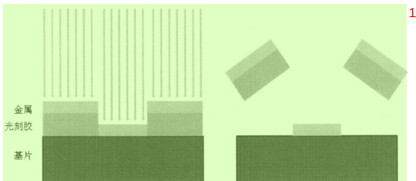
图 2.4 镀膜和 lift off 示意图
