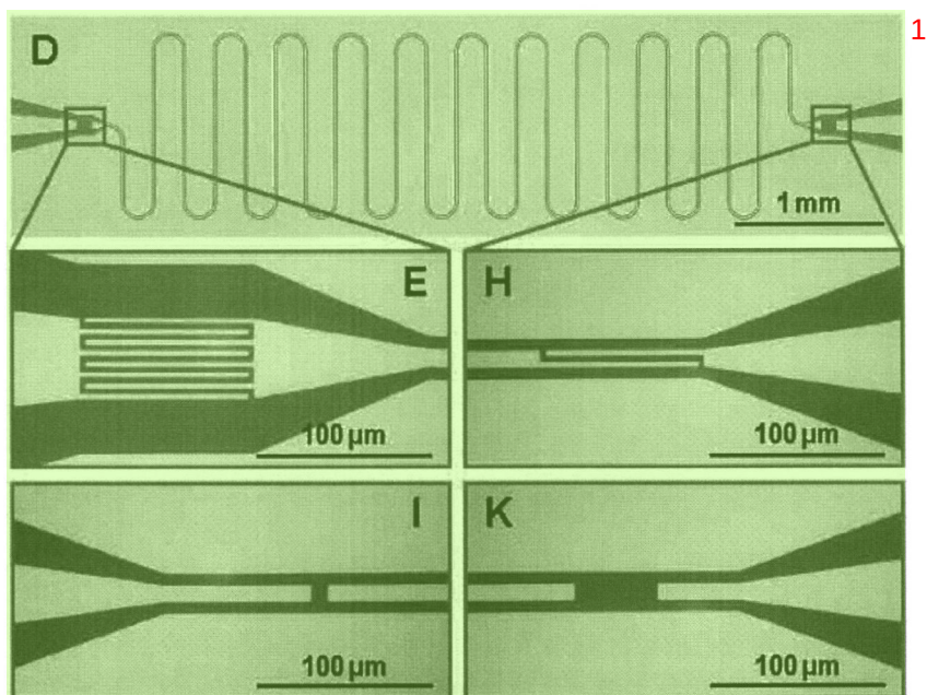
图 3.5 透射式谐振腔样品结构 [50] 2
