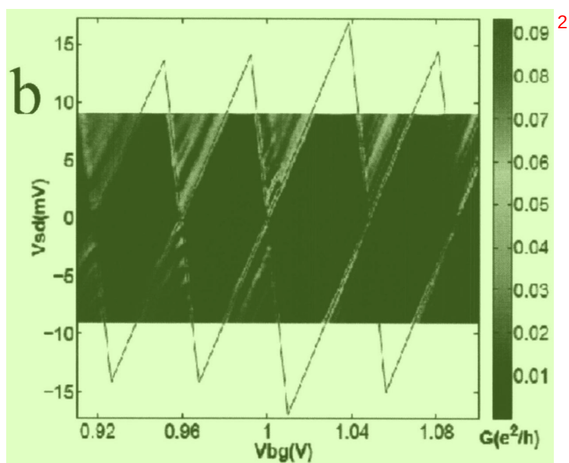
图 1.5 库伦菱形 (a) 理论 (b) 实验 [19]
