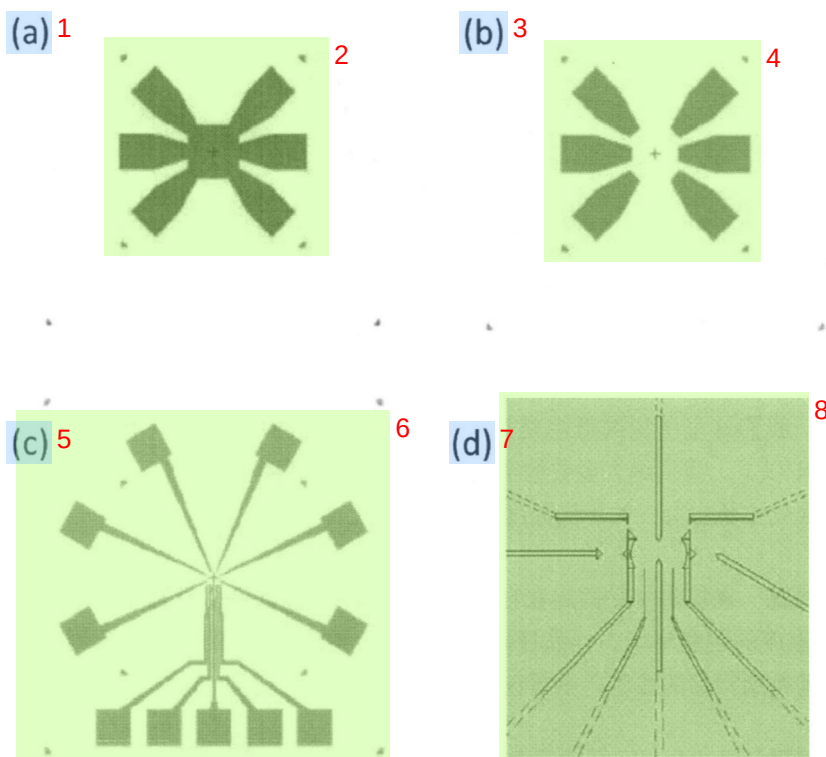
图 2.7 (a) mesa 光学曝光掩膜 (b) 欧姆电极光学曝光掩膜 (c) 表面大电极光学曝光掩膜 (d) 内部小电极 NPGS 设计图样
