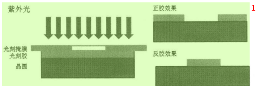
图 2.1 光学曝光正反胶示意图
