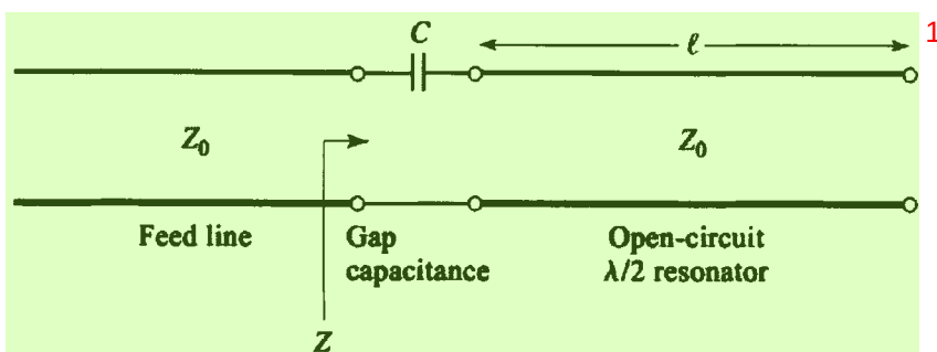
图 3.14 谐振腔和耦合缝隙的等效电路 [48] 2
