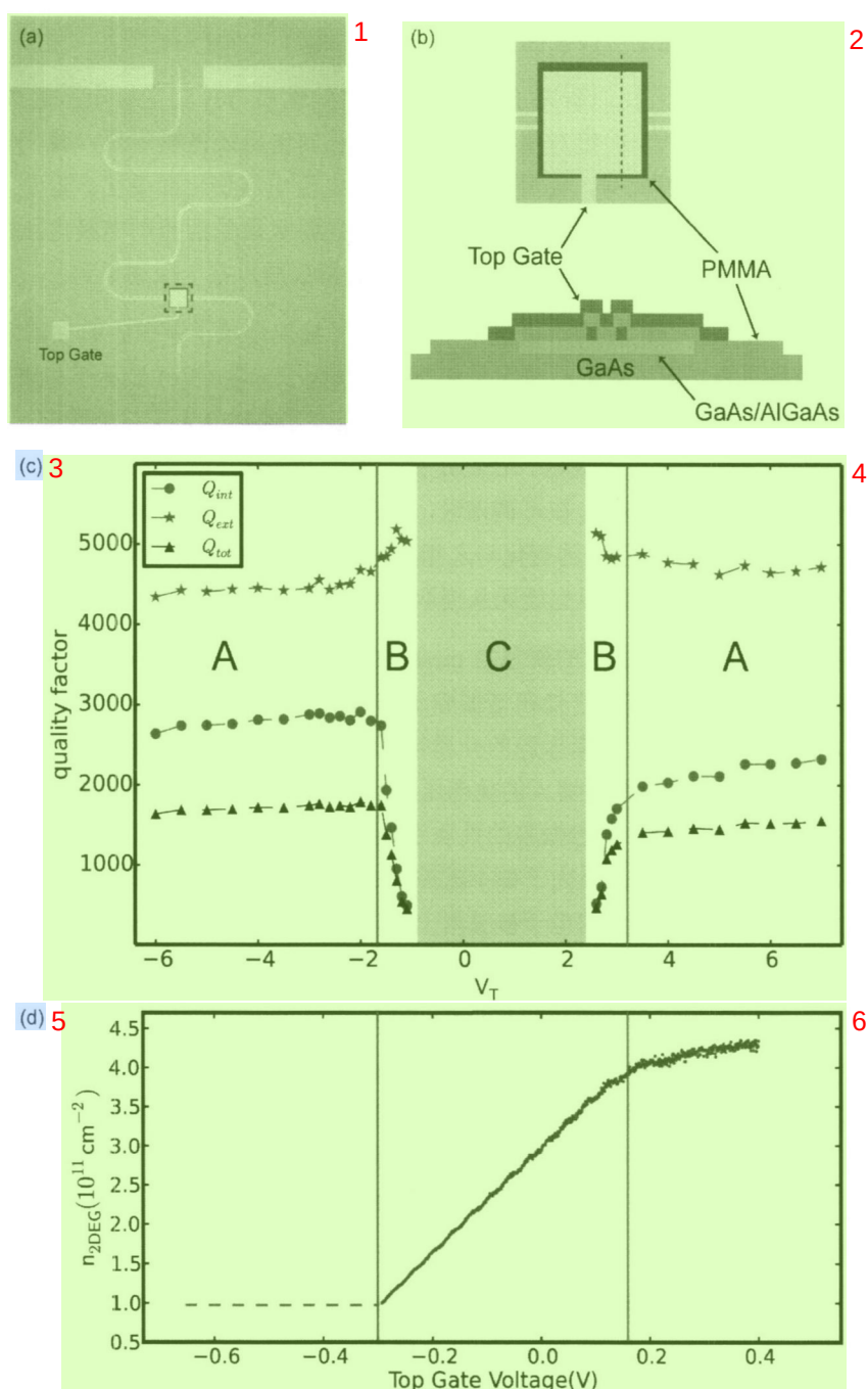
图 4.3 (a) 耦合了二维电子气的反射式谐振腔光镜图像。(b) 包含二维电子气层、PMMA 层和顶部控制门电极的谐振腔横截面。(c) 三种不同电压区域下内部品质因子（红圈）、外部品质因子（蓝星）和总的有载品质因子（黑三角）的变化：（A）稳定器，（B）可调谐区，（C）消失区。(d) 采用同样晶圆制作的 Hall bar 中电子气浓度随顶部控制电极的变化（无 PMMA 层）
