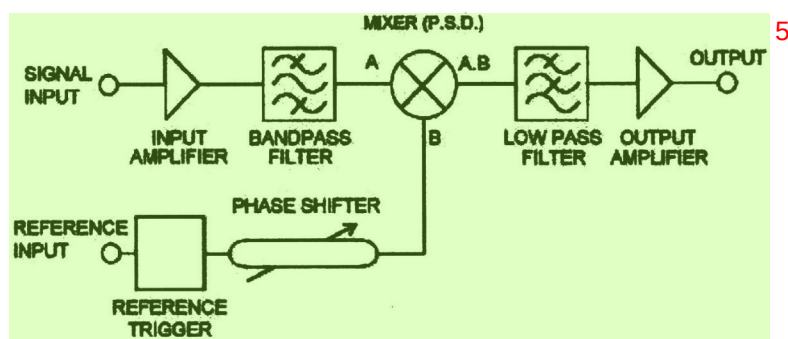
图 2.14 锁相放大器原理示意图
