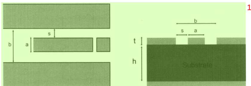
图 3.4 共面波导结构示意图 [49]
