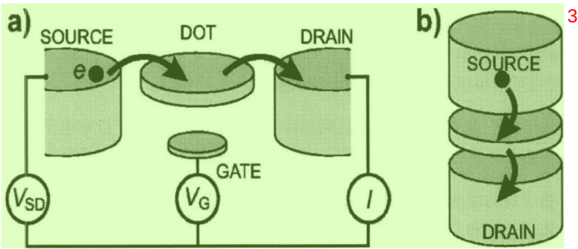
图 1.2 (a) 横向量子点 (b) 纵向量子点 [15]
