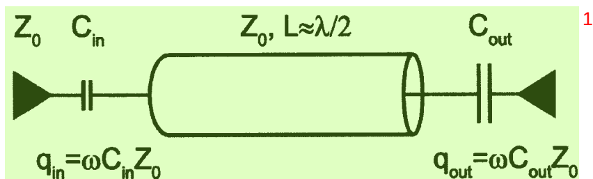
图 3.8 透射式谐振腔等效模型
