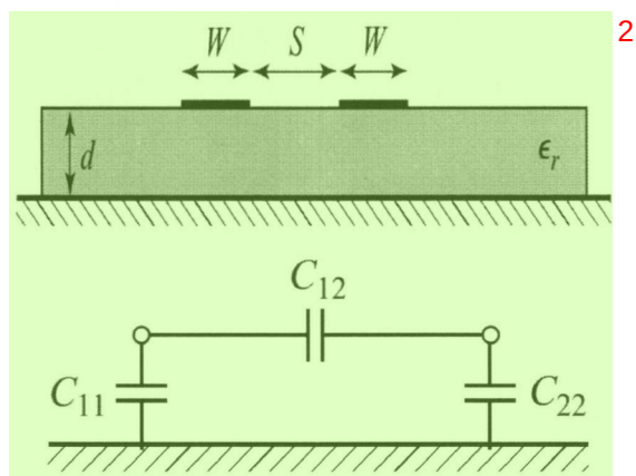
图 3.12 耦合微带线截面示意图和电容模型 [48]
