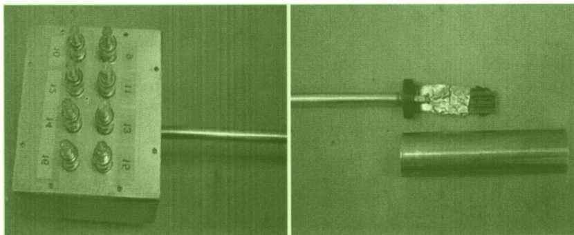
图 2.8 液氮杜瓦样品杆 2
