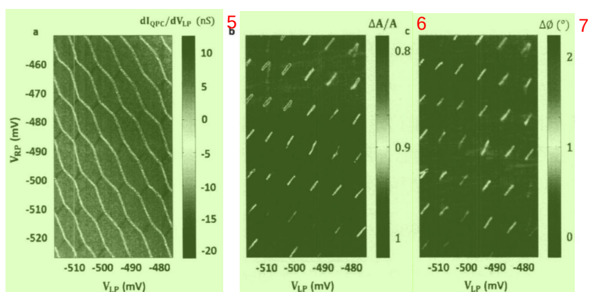
图 6.7 Graphene 双量子点电荷稳态相图 (a) 使用 QPC 调制测量 (b) 同样电压扫描区域谐振腔振幅变化信号 (c) 谐振腔相位变化信号 8
