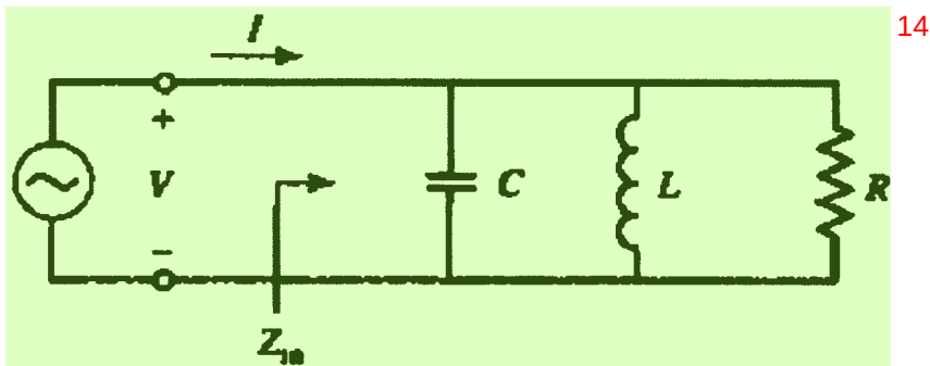
图 3.1 集总并联谐振电路示意图 [48] 15
