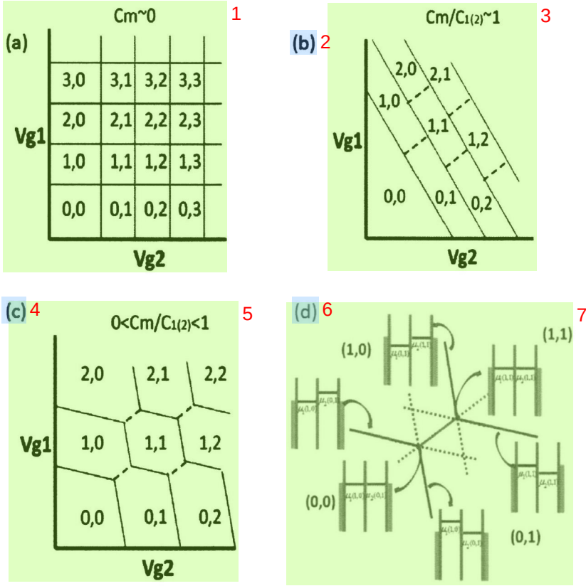
图 1.7 双量子点蜂窝相图 (a) 弱耦合 (b) 强耦合 (c) 中等耦合 (d) 量子点能级分布的变化 8
