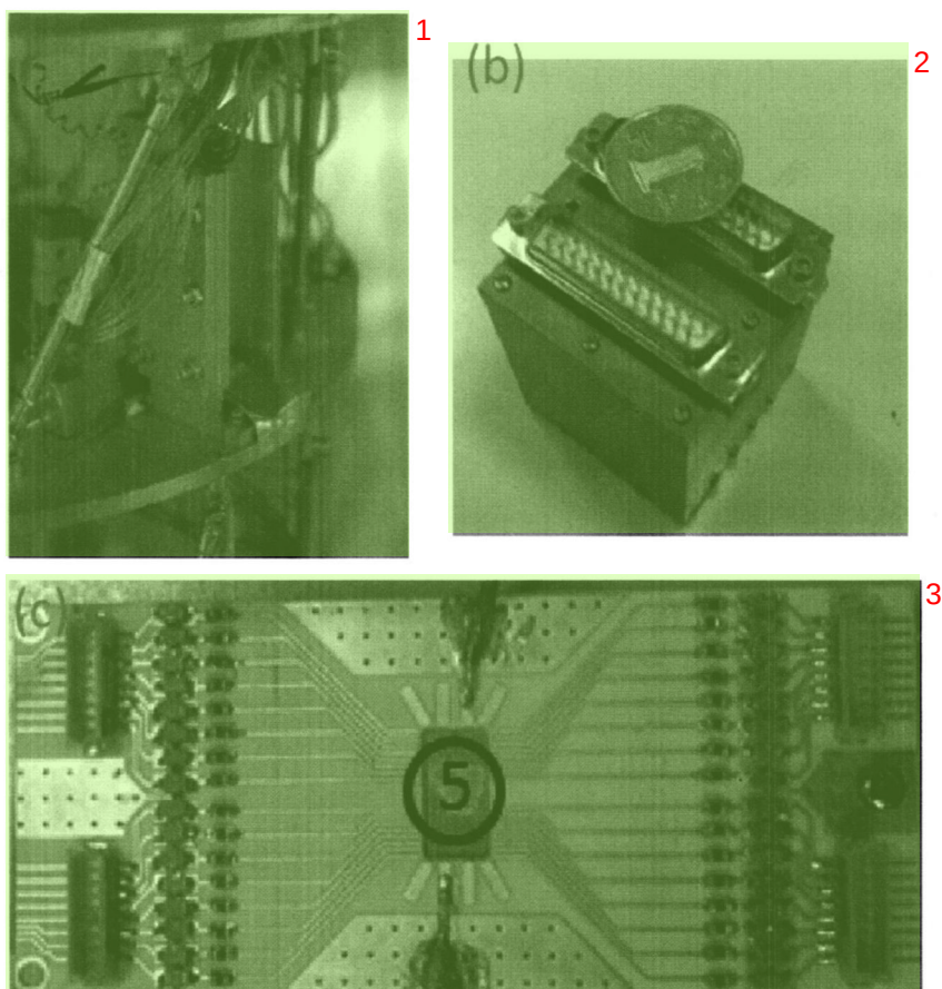
图 2.13 (a) 多层夹板式热沉 (b) 铜粉滤波器 (c) 装有铁氧体磁珠低通滤波器的 PCB chip carrier
