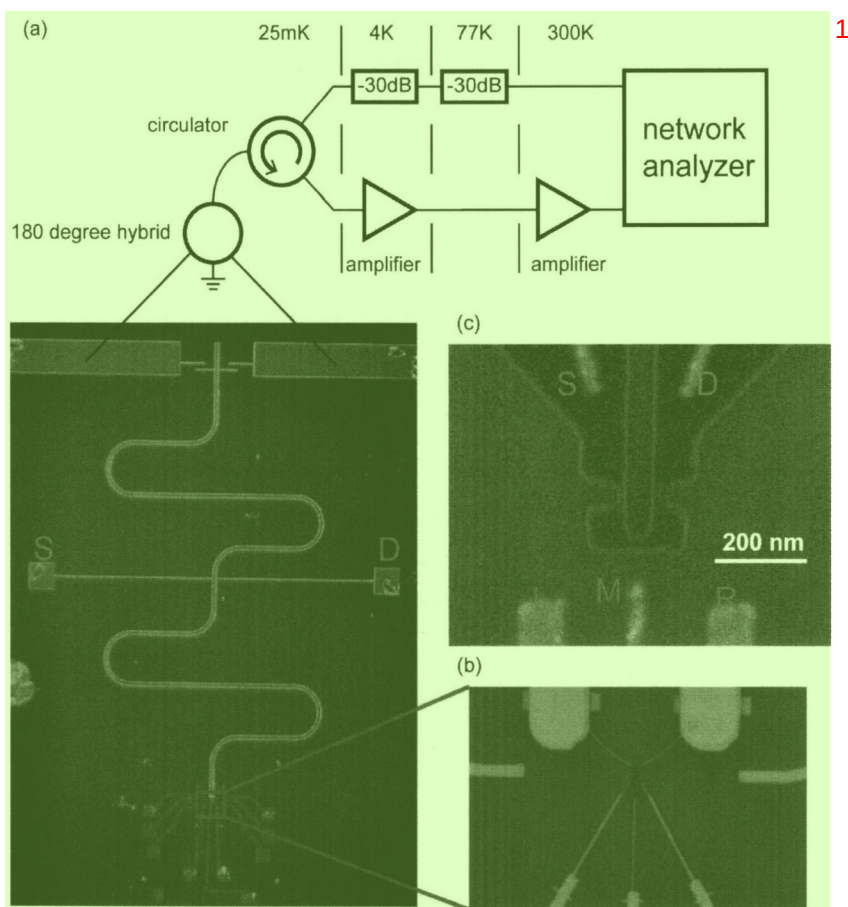
图 5.1 (a) 反射式谐振腔和 Graphene 量子点耦合结构在光学显微镜下的图像，以及微波测量电路示意图 (b) 量子点附近放大图像 (c) 量子点电子显微镜成像。黑色区域为 Graphene 结构。量子点连接谐振腔的电极为 S 和 D，门控制电极为 L、M 和 R。
