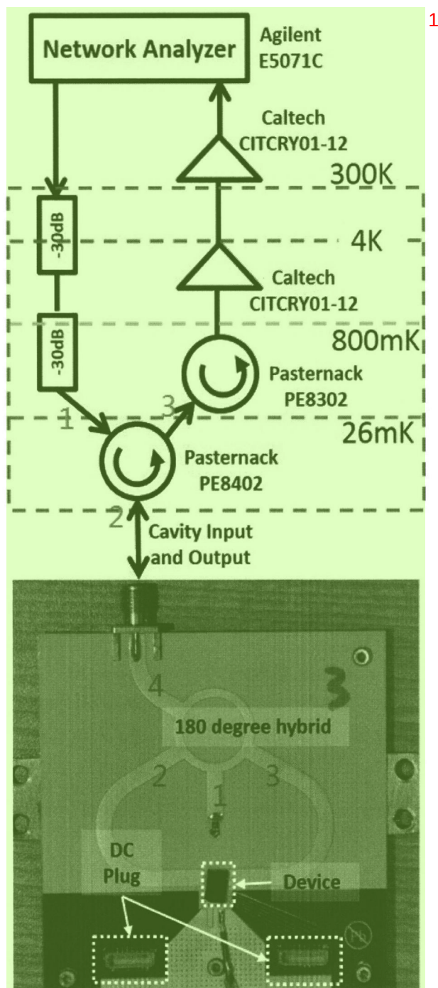
图 3.17 反射式谐振腔测量电路
