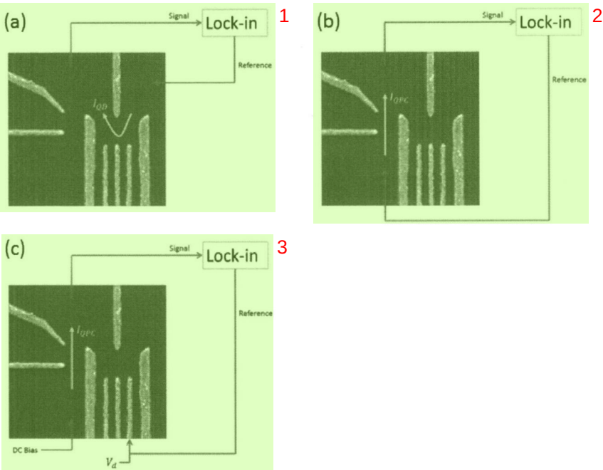
图 2.15 三种不同的 lock-in 测量方式。(a) 量子点输运信号测量 (b)QPC 输运信号测量 (c)QPC 调制信号测量
