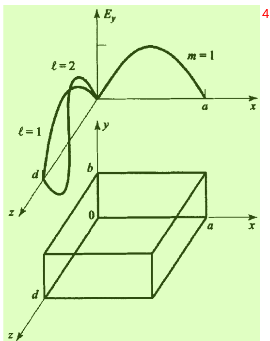
图 3.20 矩形谐振腔 [48]
