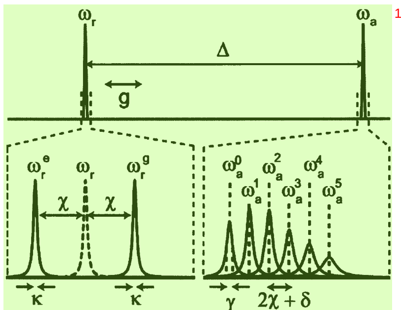
图 6.2 强色散区中原子和光子的能谱 [49]。2
