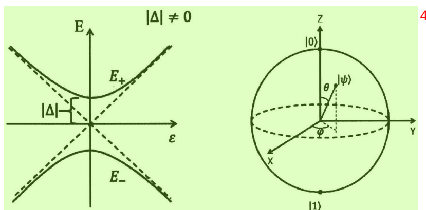
图 1.9 二能级结构和 Bloch 波矢 [13]
