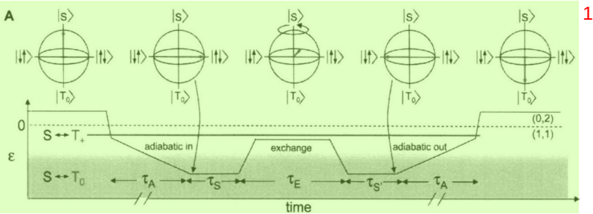
图 1.10 Rabi 振荡中 Bloch 波矢的演化 [26] 2
