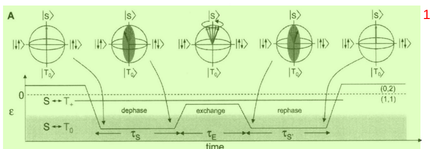
图 1.12 Echo 技术中 Bloch 波矢的演化 [26] 2
