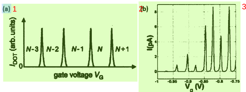
图 1.4 库伦振荡 (a) 理论 (b) 实验
