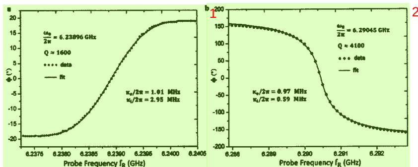
图 3.15 透射式谐振腔相位随频率的变化
